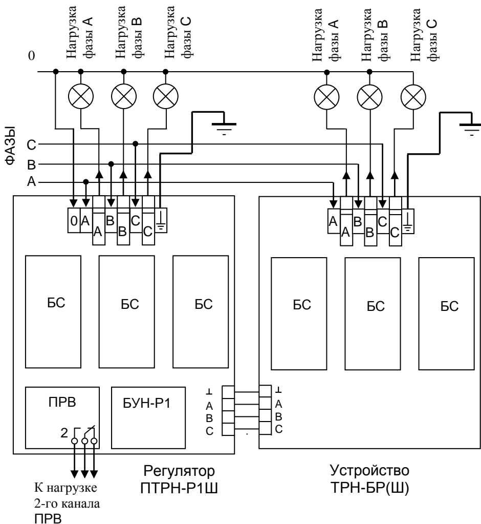
СХЕМА СОЕДИНЕНИЙ
